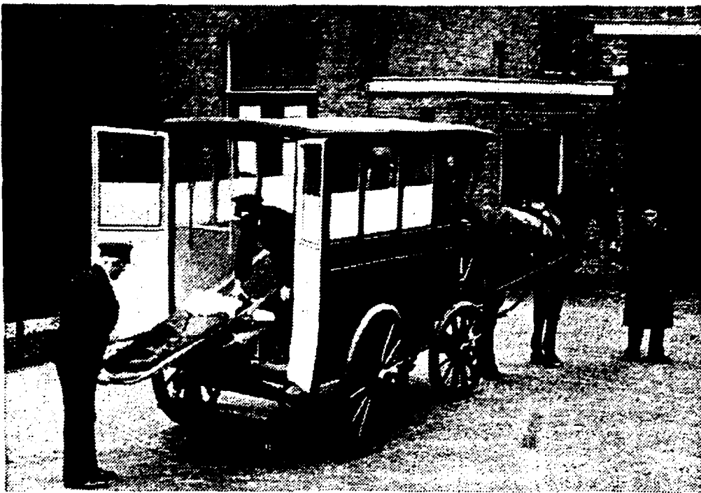
Ter besparing van benzine is de Gem. Geneeskundige Dienst in Den Haag er toe overgegaan het vervoer van zieken van minder ernstigen aard per paard en wagen te doen geschieden. De wagen is praktisch ingericht, en is voorzien van wielen met gummibanden.
